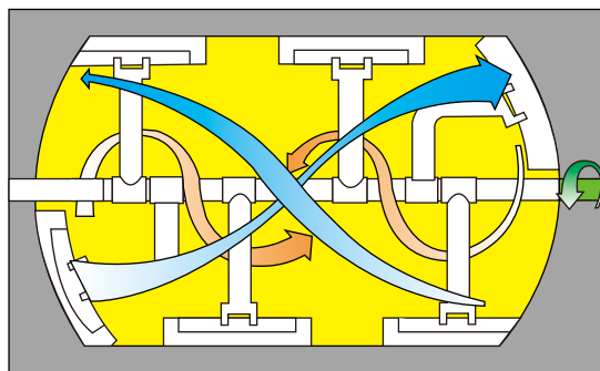
"S"型刮壁设计，避免物料粘锅
